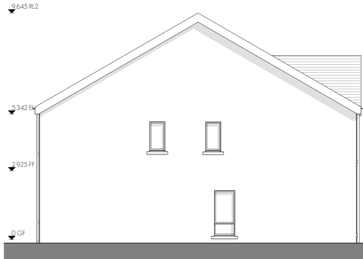
SIDE ELEVATION A1 1:100
