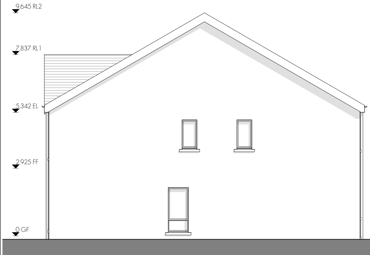
SIDE ELEVATION A1 1:100
